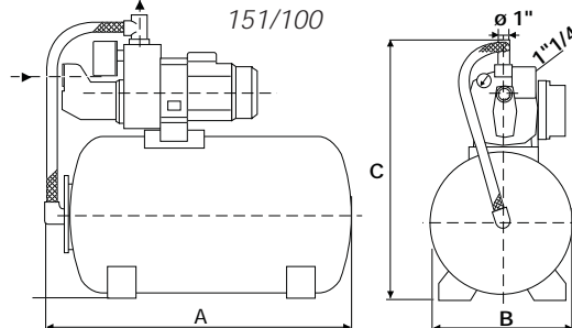
AQUAJET 132/100 151/100
