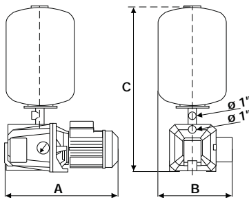
AQUAJET 102/-60-80
